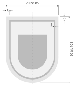
Abb. 4 – Maße Ärmelabzeichen
